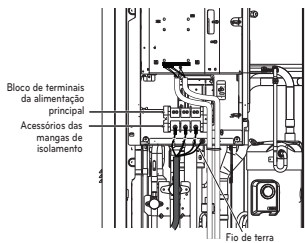
Ligação da linha de alimentação principal
