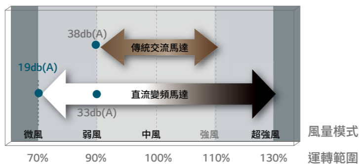
室內機風扇風量可變範圍
